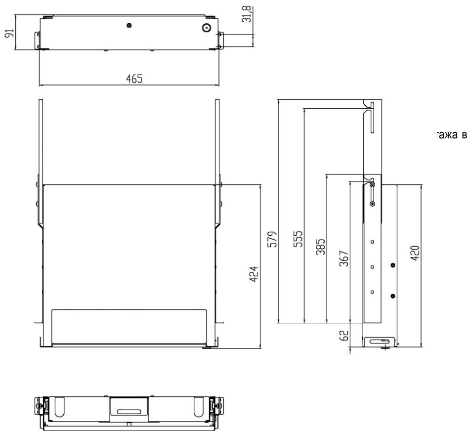
Рисунок 5: Монтажно-габаритный чертеж REC-SVMT-C
